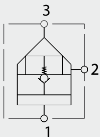
Schaltzeichen »modern« nach DIN 24342
